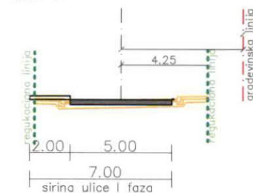
presjek E-E
