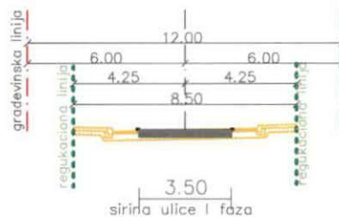
presjek O-O
