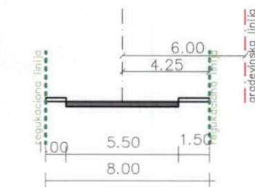
presjek E-E
